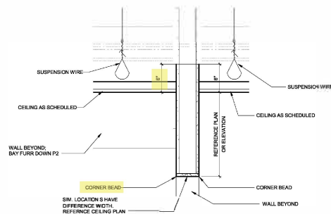
2 CEILING DETAIL SCALE: 1/8" = 1'-0"
