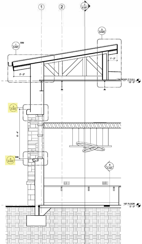
5 WALL SECTION SCALE: 1/2" = 1'-0"
