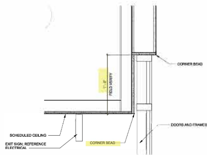
1 CEILING DETAIL SCALE: 1/8" = 1'-0"
