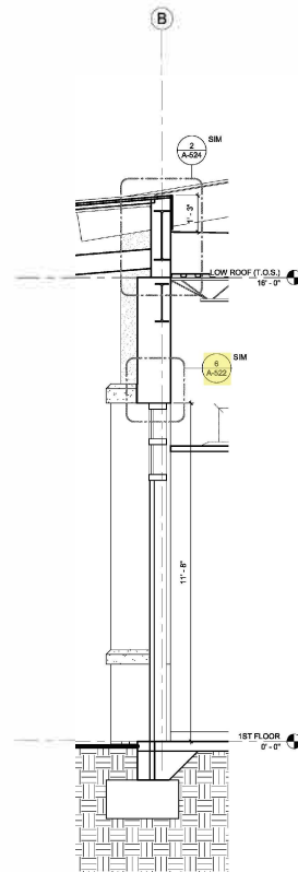
4 WALL SECTION SCALE: 1/2" = 1'-0"
