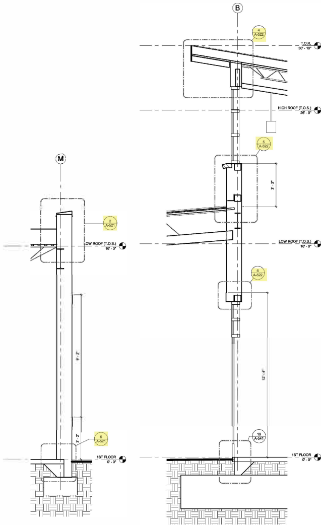
1 WALL SECTION SCALE: 1/2" = 1'-0"
