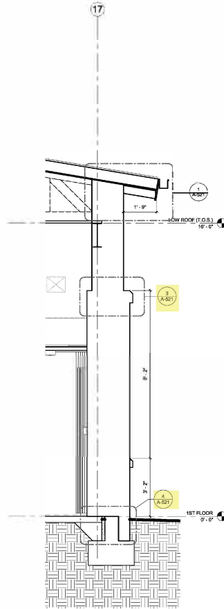
3 WALL SECTION SCALE: 1/2" = 1'-0"
