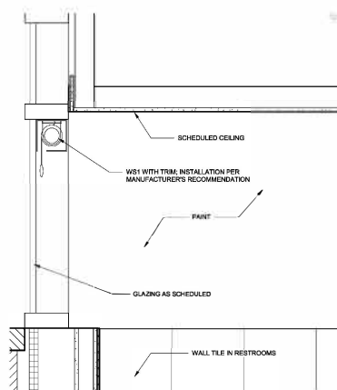
4 CEILING DETAIL SCALE: 1/8" = 1'-0"
